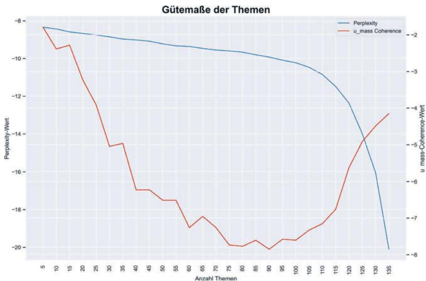
Abbildung 11.5 Coherence- und Perplexity-Scores für 5 bis 135 Themen
