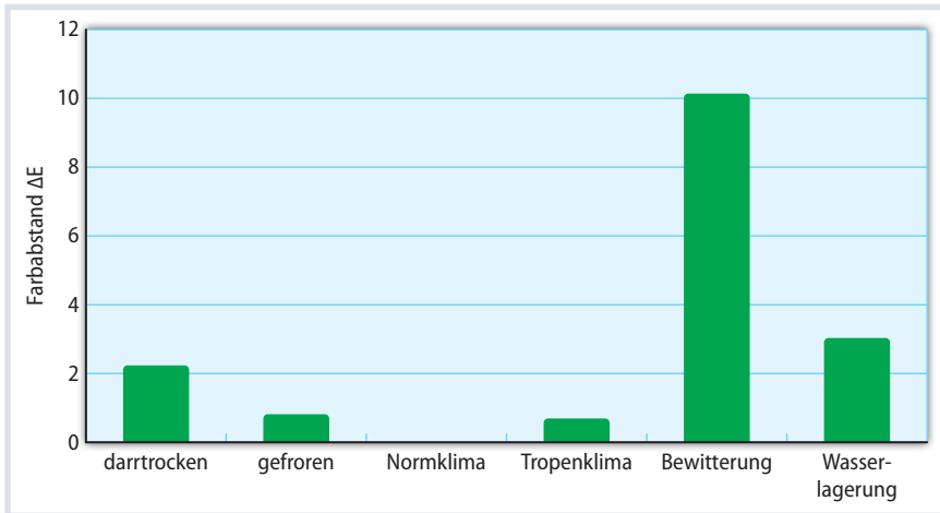
Bild 6. Farbabstand der verschiedenen konditionierten Proben bezogen auf die Farbe bei Normklima: Die größte Farbabweichung ist bei der bewitterten Probe festzustellen. Bei den verschiedenen Trockenverfahren kommt es bei der Darrtrocknung zur größten Abweichung.
