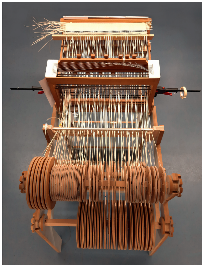
Bild 2. Für die Verarbeitung von Weidenfäden zu Geweben wurde ein Webstuhl entsprechend umgebaut. © FBKE
