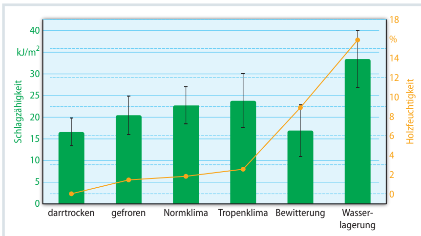
Bild 7. Feuchtigkeit und Schlagzähigkeit der konditionierten Prüfkörper: Die Schlagzähigkeit nimmt besonders nach der Wasserlagerung deutlich zu. Quelle: XXXXXXXXXX; Grafik: © Hanser
