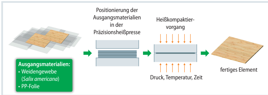
Bild 3. Im Heißkompaktierverfahren werden mehrere Lagen der PP-Folie mit den Weidengeweben verbunden. Quelle: XXXXXXXXXX; Grafik: © Hanser
